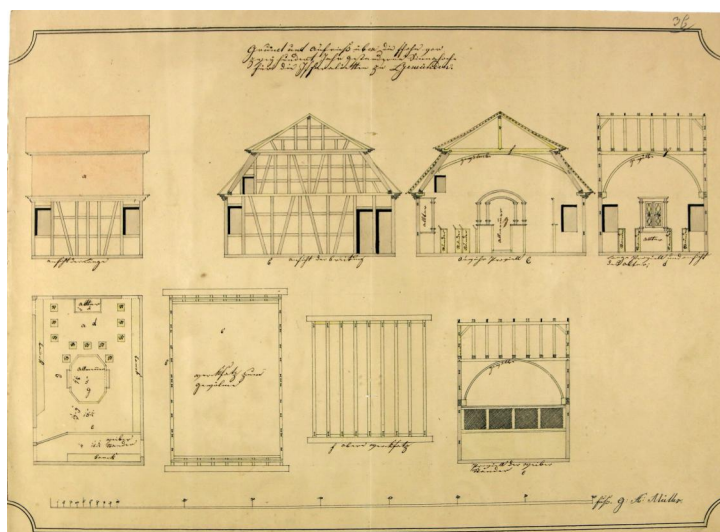
Vermutlich nach Vorlage eines barocken Bauplans 1838 angefertigte Bestandsaufnahme der Synagoge zu Gemünden. Mit diesem "Grund und Aufriß über die schon vor zwey hundert Jahr gestandene Sinnachoche für die Isseralietten zu Gemünden" konnte die Gemeinde gegen die Kreisregierung den Fortbestand der Synagoge erreichen. Copyright Staatsarchiv Würzburg (Regierung von Unterfranken 8466, fol. 35 f.)
