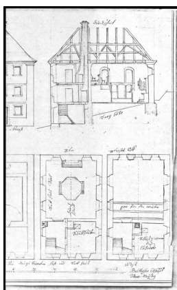
Heiligenstadt, Plan des Synagogengrundstücks mit Grund- und Aufriss sowie einem Querschnitt des Synagogen-Neubaus (Maurermeister Balthasar Haupt, 15. Januar 1819). Copyright Universitätsarchiv Bamberg, Forschungsstelle Landjudentum (Prof. Klaus Guth, Signatur 102/Heiligenstadt/00002-04).
