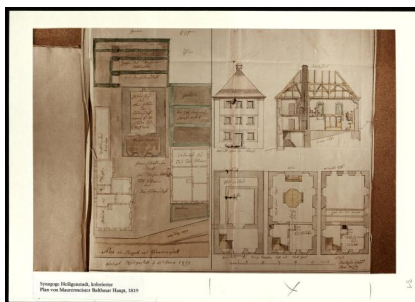
Heiligenstadt, Plan des Synagogengrundstücks mit Grund- und Aufriss sowie einem Querschnitt des Synagogen-Neubaus (Maurermeister Balthasar Haupt, 15. Januar 1819). Copyright Universitätsarchiv Bamberg, Forschungsstelle Landjudentum (Prof. Klaus Guth, Signatur 102/Heiligenstadt/00002-04).
